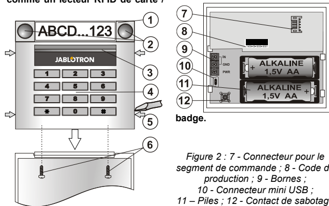
Figure 1 : 1 - Segment de commande ; 2 - Touches du segment ; 3 - Touche rétro-éclairée d'activation ; 4 - Module d'accès avec lecteur RFID ; 5 - Languette pour l'ouverture du module ; 6 - Vis du capot
